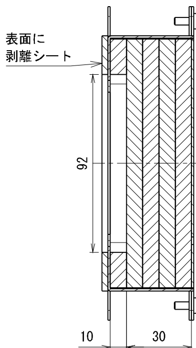
断面 A-A
