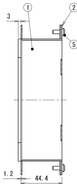
断面 A-A
